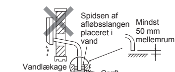
Vandlækage Grøft
